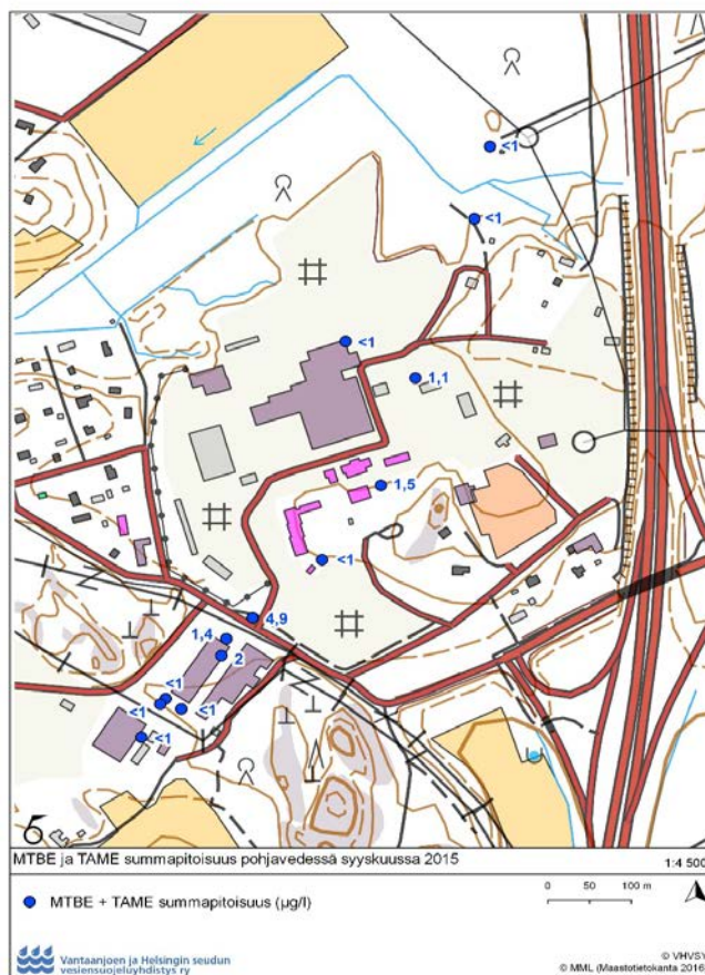
Kuva 13. Bensiinin lisäaineiden (MTBE ja TAME) summapitoisuus pohjavedessä syyskuussa 2015.
